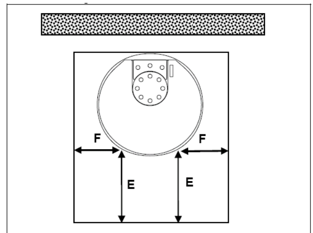
Abb. 4: Funkenschutzvorlage KK 80-1
