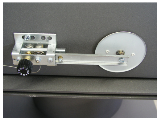
Abb. 12: Thermoregelung Stellung 0
