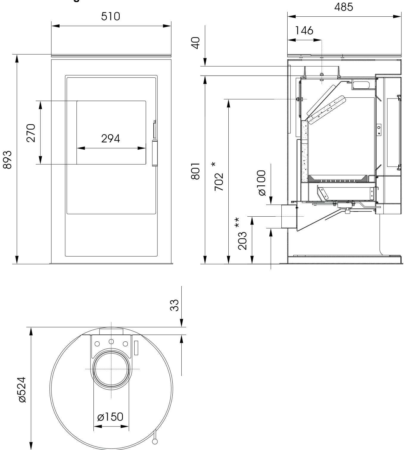
Abb. 1: Maßzeichnung KK 80-1
