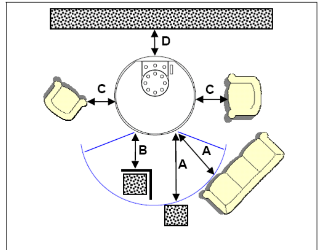
Abb. 3: Brandschutzabstände KK 80-1
