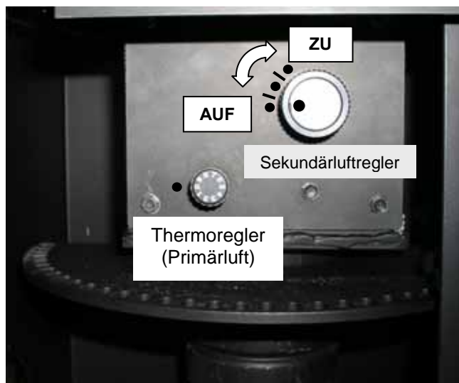
Abb. 27: Einstellung Thermoregler und Sekundärluftregler
