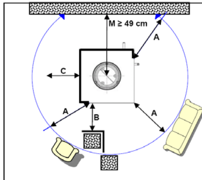
Abb. 4: Brandschutzabstände Ofen gerade
