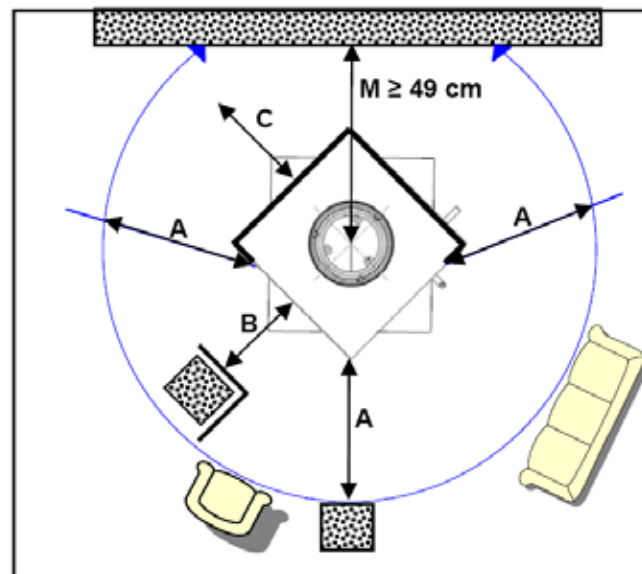
Abb. 5: Brandschutzabstände Ofen gedreht
