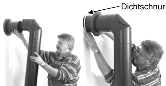
Abb. 20: Anschluss Rauchrohr am Schornstein
