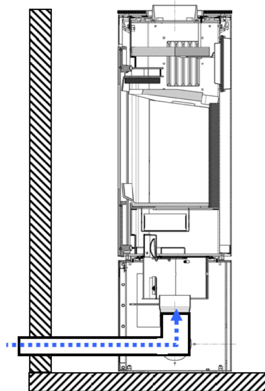
Abb. 18: Vom Nebenraum oder über separaten Luftschacht
