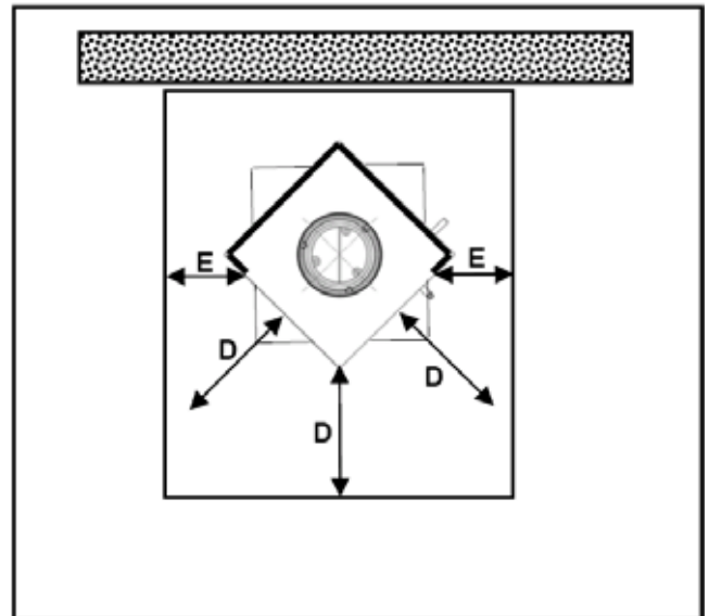
Abb. 7: Funkenschutzvorlage – Ofen gedreht
