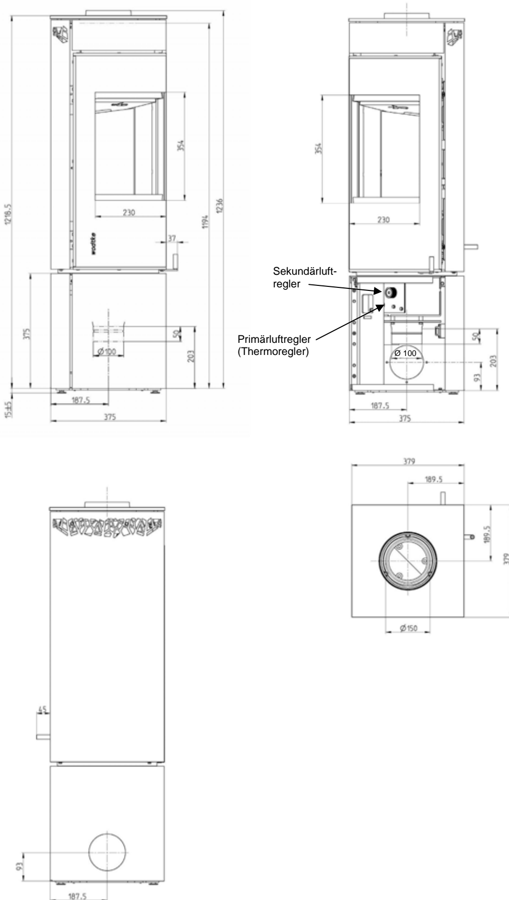
Abb. 1: Maßzeichnung KK 95
