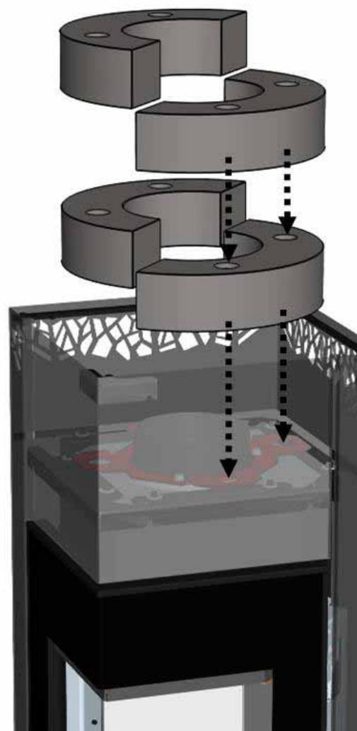
Abb. 13: Einsetzen der wotdke Speichersteine (nur KK95-1)
