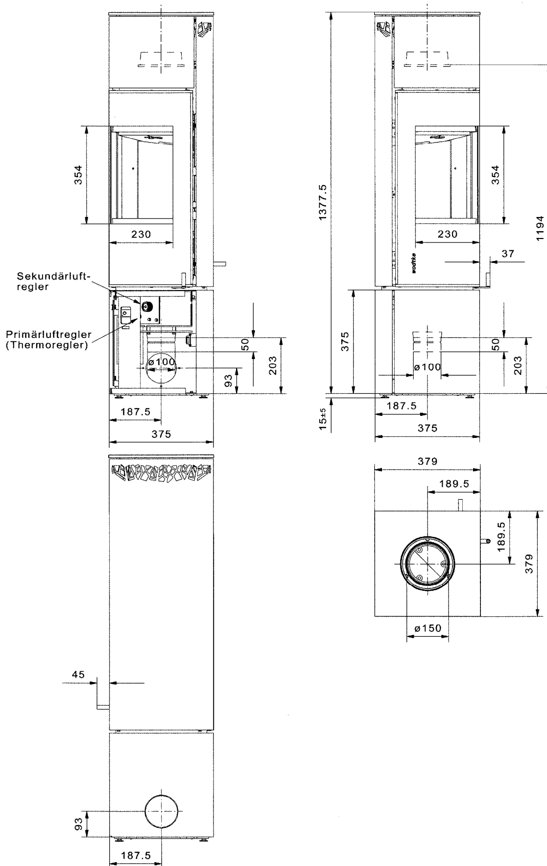
Abb. 2: Maßzeichnung KK 95-1
