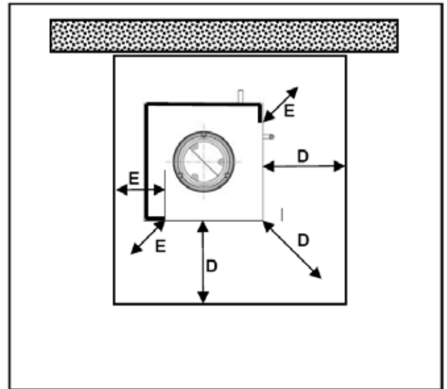
Abb. 6: Funkenschutzvorlage – Ofen gerade
