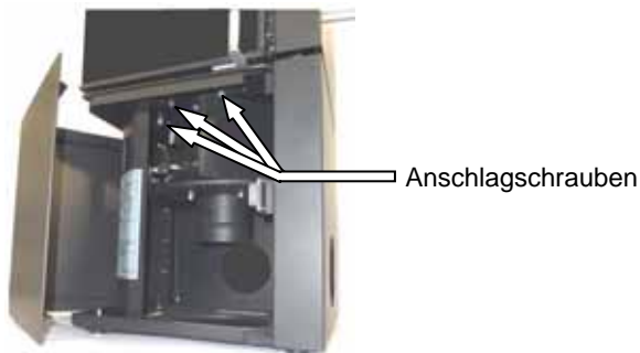
Abb. 8: Position Anschlagsschrauben
