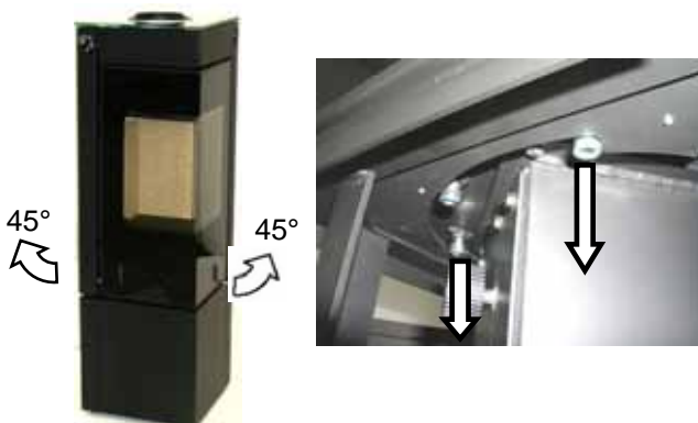
Abb. 9: Schwenkbereich \pm 45^\circ nach links und rechts
