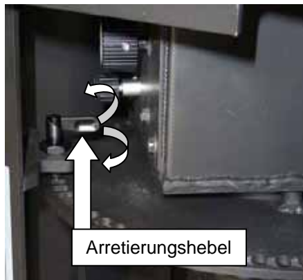
Abb. 24: Arretierungshebel Schwenkvorrichtung
