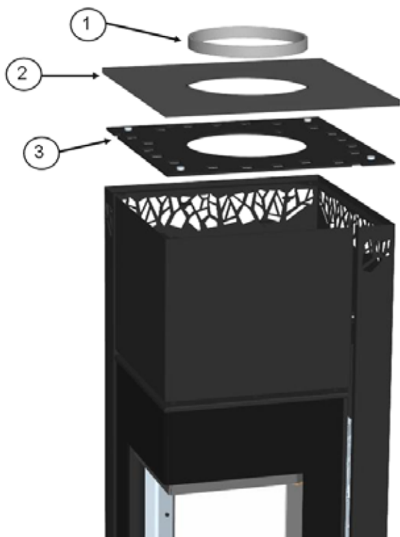
Abb. 12: Entfernen oberer Deckel (nur KK95-1)
