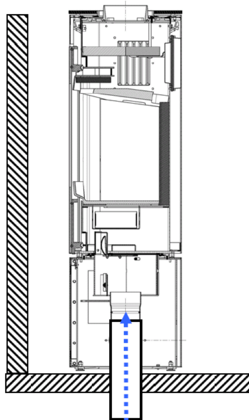
Abb. 17: Von unten Keller / UG (Empfehlung)
