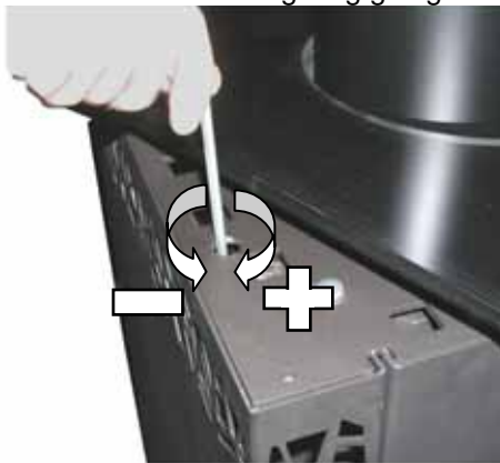
Abb. 22: Einstellen Türvorspannung
