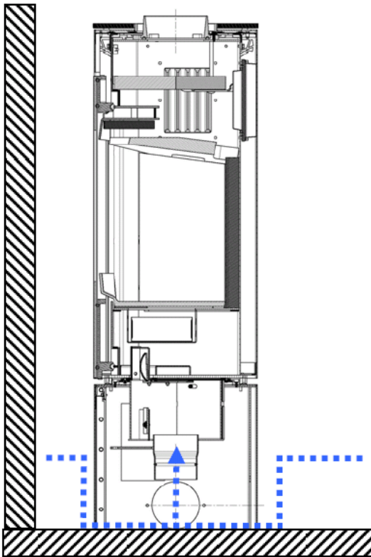
Abb. 16: Ansaugung aus dem Aufstellraum
