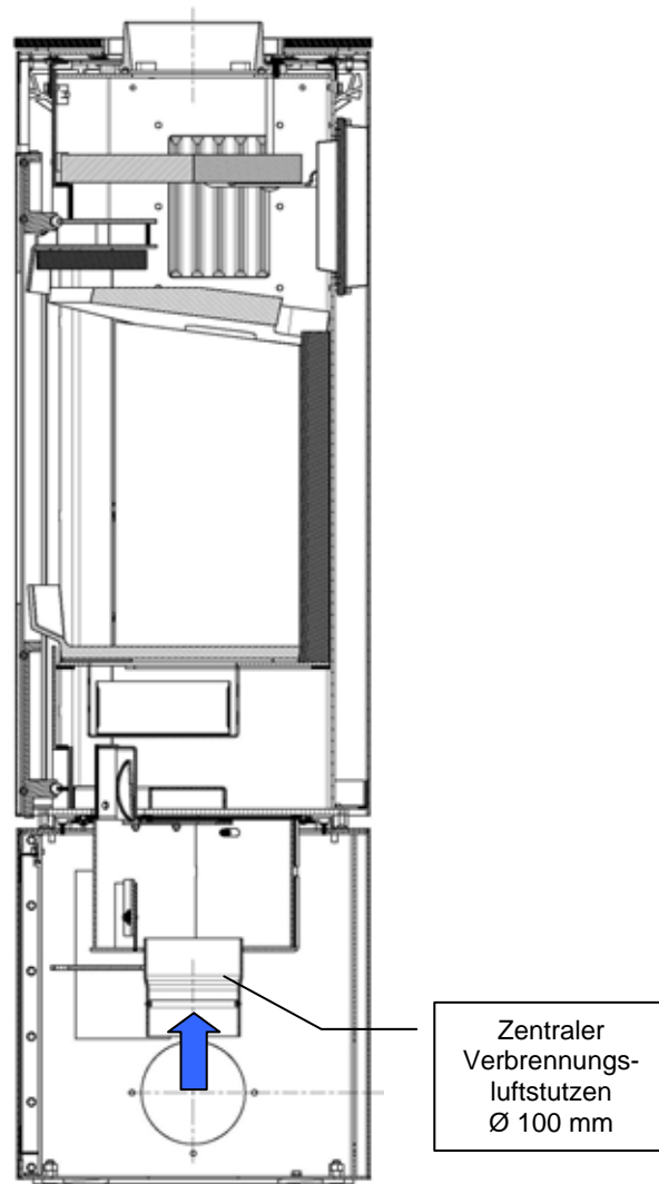
Abb. 15: Zentraler Verbrennungsluftstutzen (Schnittbild)
