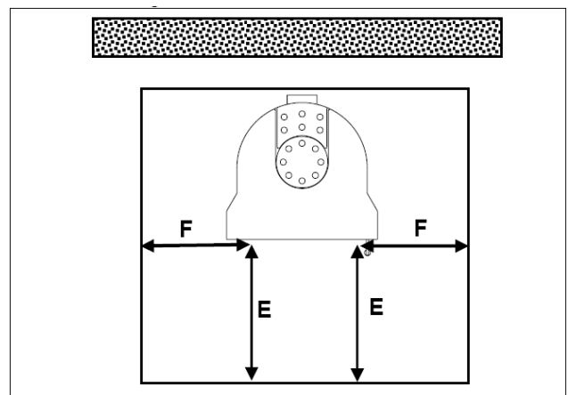
Abb. 4: Funkenschutzvorlage KK 80-2
