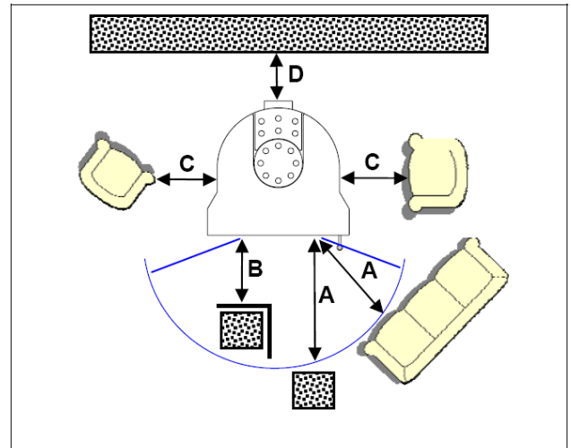
Abb. 3: Brandschutzabstände KK 80-2
