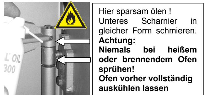
Abbildung 19: Ölen Türscharnier
