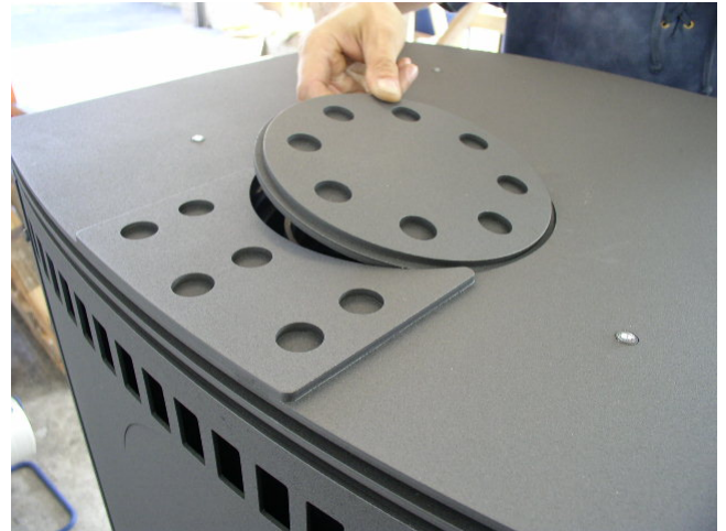
Abbildung 7: Abdeckung Rauchrohranschluss
