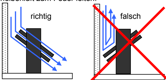
Abbildung 6: Position Stehrost
