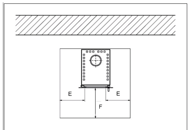
Abb. 6: Funkenschutzbürzel KK 20
