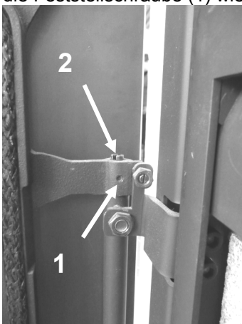
Abb. 11: Türfederspannung nachstellen
