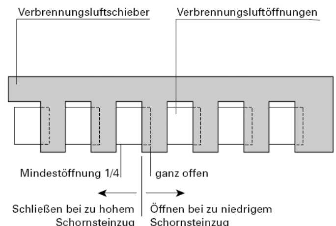
Abb. 13: Anpassen Verbrennungsluftquerschnitt
