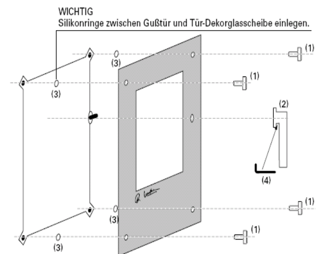
Abb. 8: Montage Dekorglas
