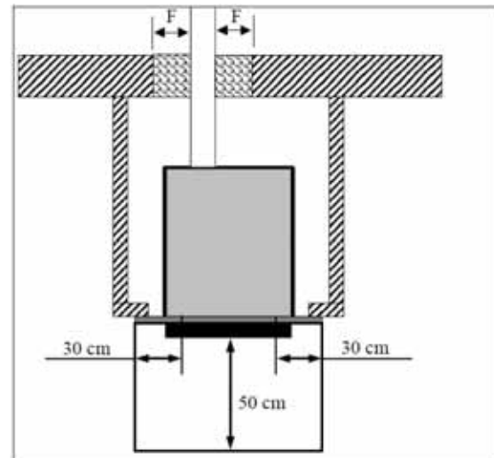
Beispiel mit Verbindungsstück durch Außenwand
