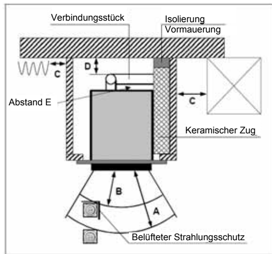
Beispiel mit Verbindungsstück zu keramischem Zug
