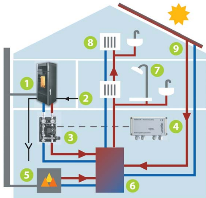
Der Anschluss an CO 2 -neutrales Heizen mit Holz — wodtke Kaminöfen water+
