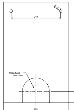
Wandkonsole "ROCKY" Rückansicht (Bohrbild)
