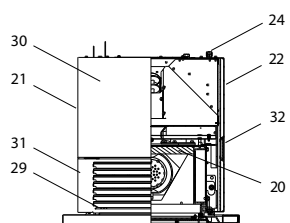
Brennertopf-Ausführung mit Auflage
