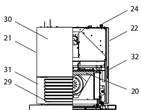
Brennertopf-Ausführung mit Auflage
