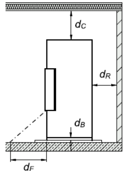
Fig. 3 distances de sécurité
