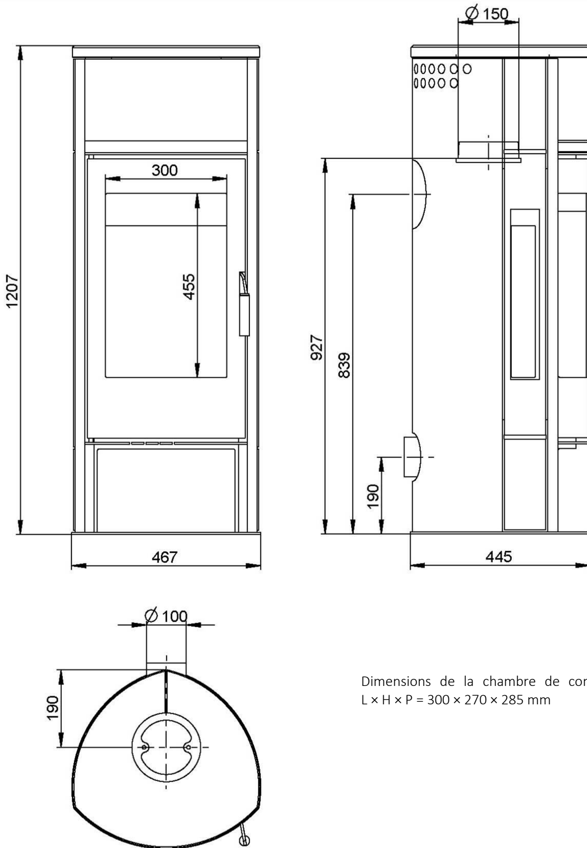
Fig. 1 : plan coté „Lucky“
