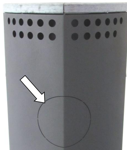
Fig. 5 : Découpe de la paroi latérale
