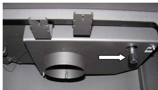
Fig. 13 : position molette de réglage du thermorégulateur
