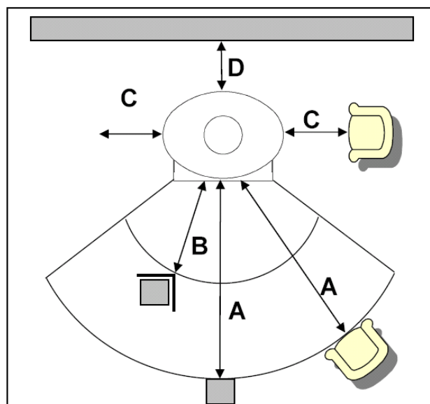
Fig. 3 : distances de sécurité K140A
