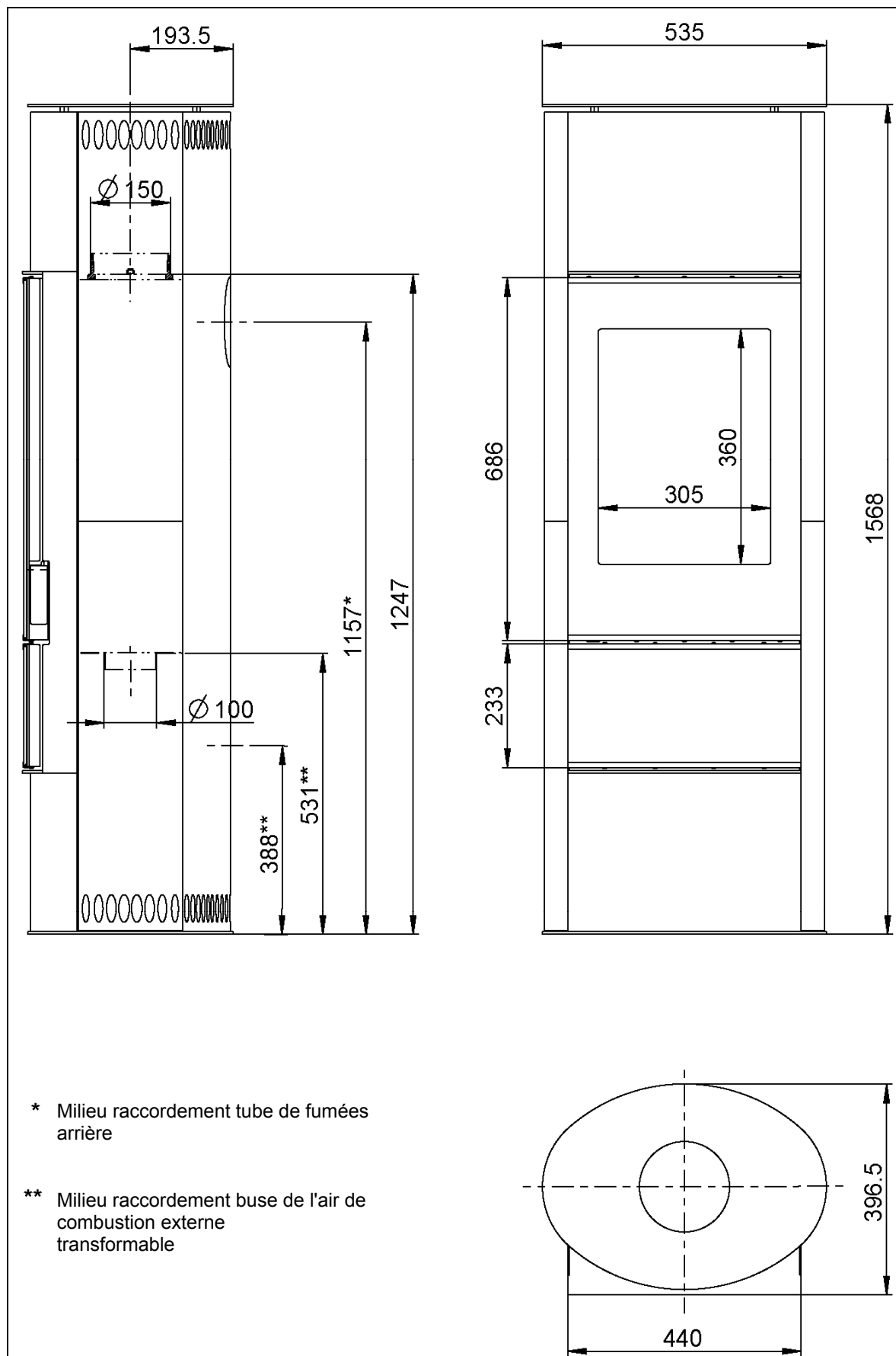
Fig. 1 : plan coté K140A
