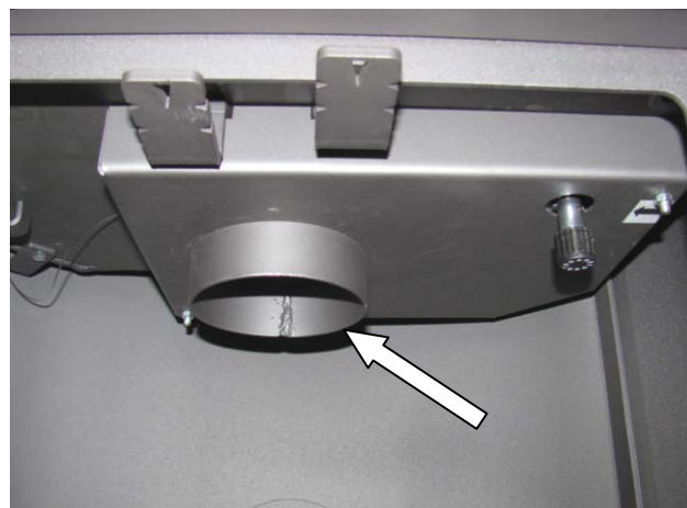
Fig. 9 : manchon d'air de combustion
