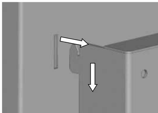
Fig. 6 : détail montage corps du poêle
