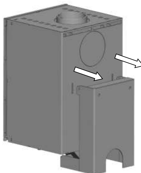
Fig. 5 : montage corps de base
