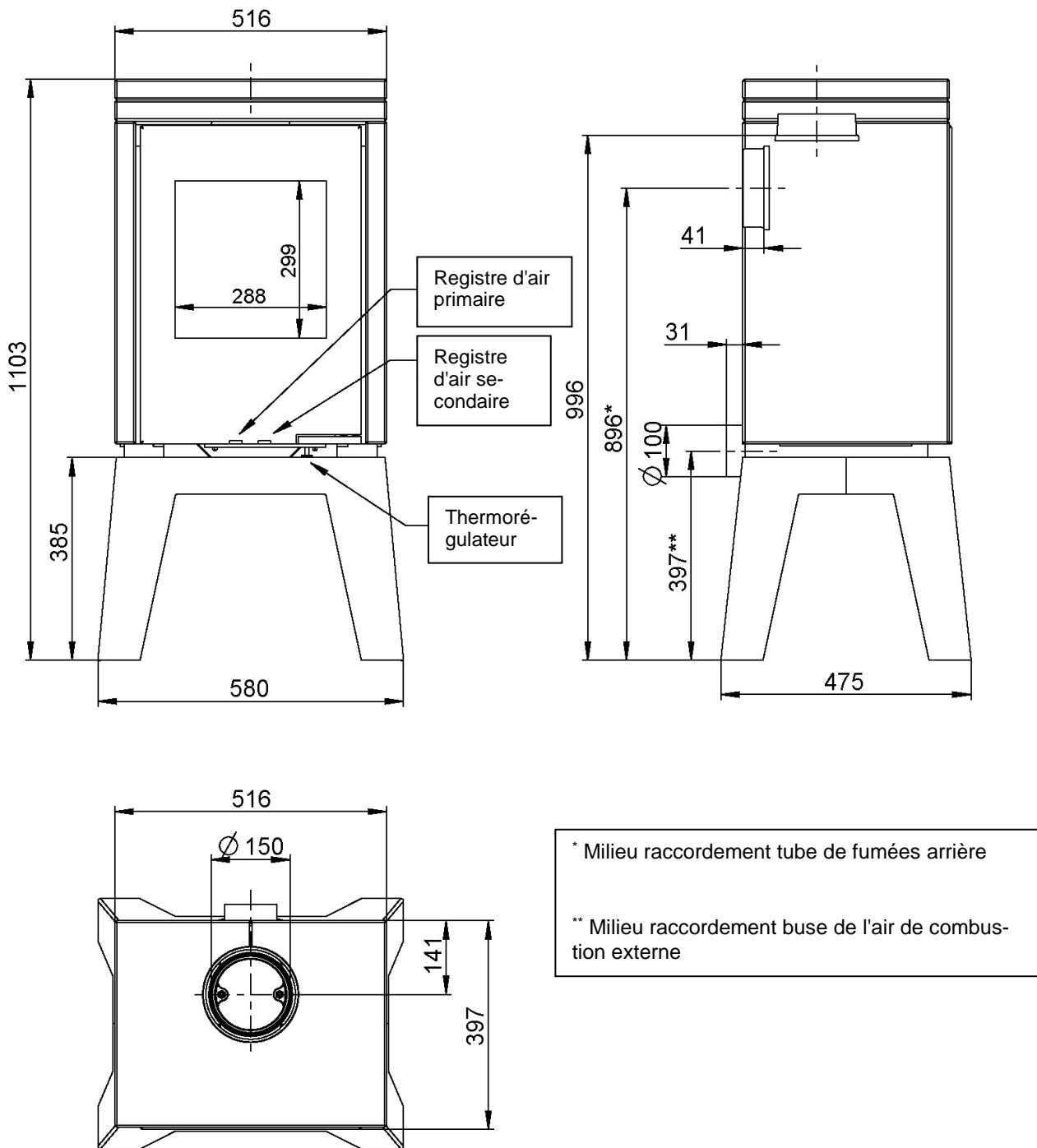
Fig. 3 : plan coté KK 80-12-4
