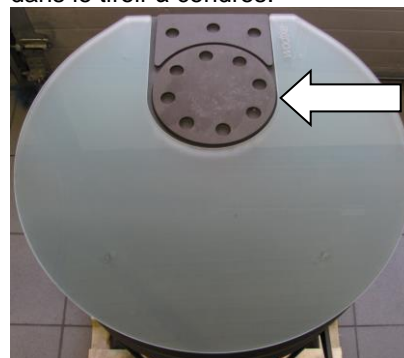
Fig. 8 : couvercle d'obturation pour le raccordement à la buse à l'exemple du Bo
