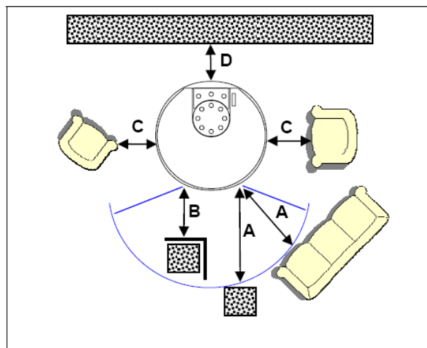
Fig. 5 : distances de sécurité KK 80-12
