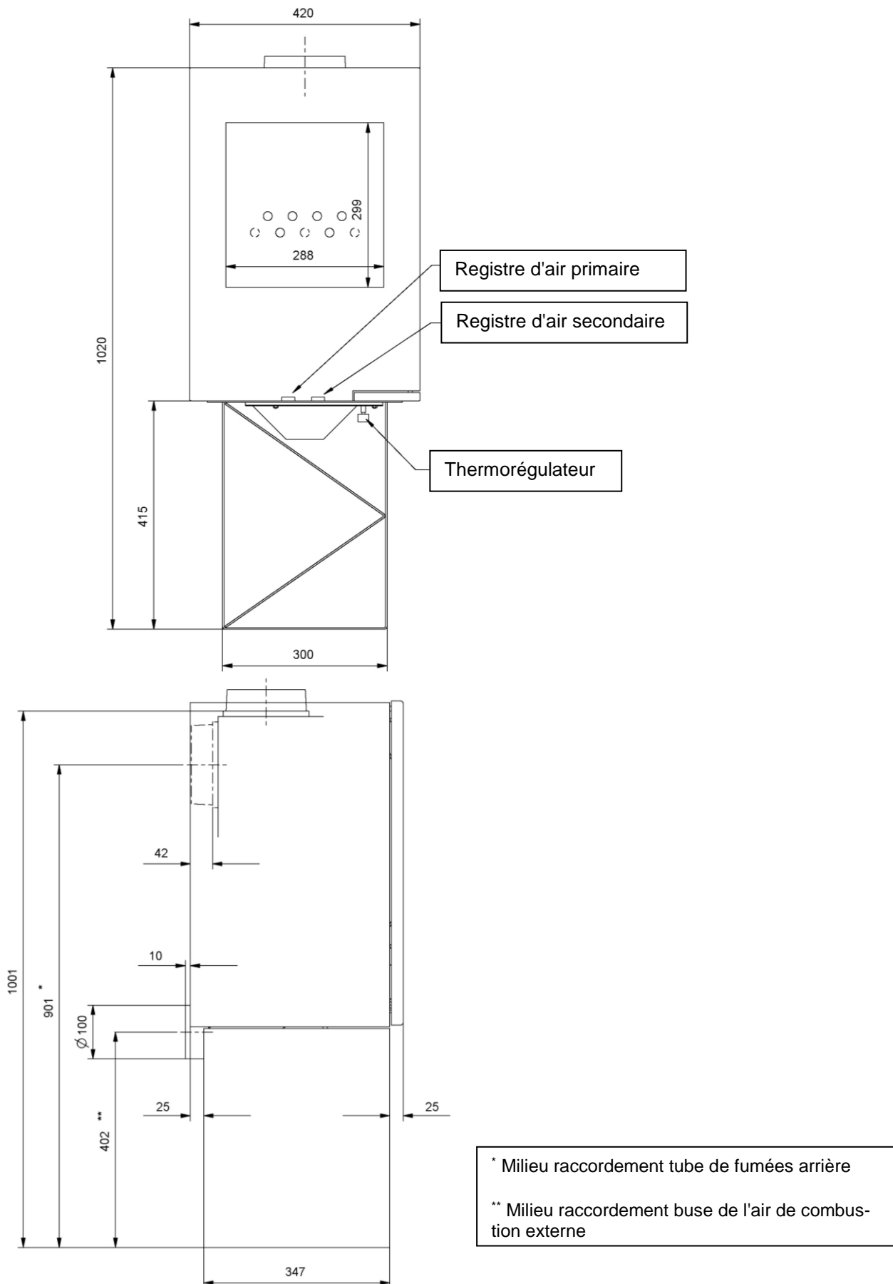
Fig. 2 : plan coté KK 80-12-3
