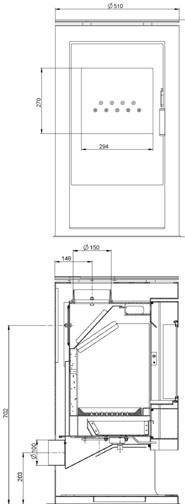
Fig. 1 : plan coté KK 80-12-1
