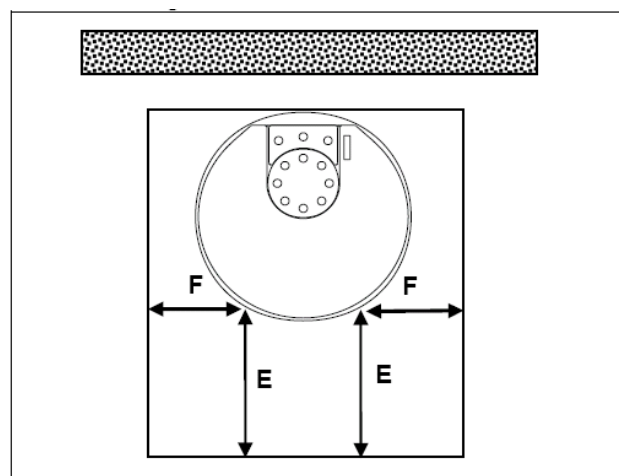
Fig. 6 : protection anti-étincelles KK 80-12
