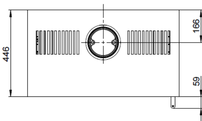
Fig. 1 : plan coté « myCastle » sans rehausse
