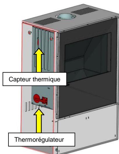
Fig. 19 : position du thermorégulateur
