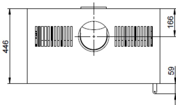
Fig. 3 : plan coté « myCastle » avec deux rehausses
