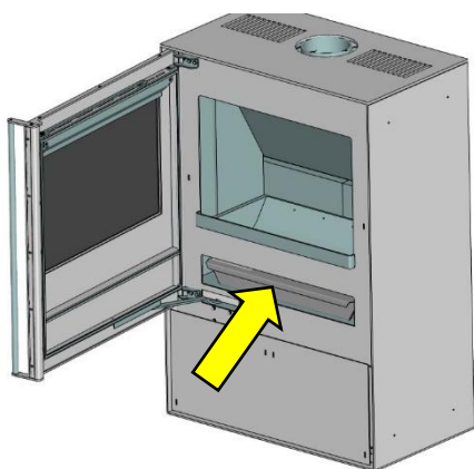
Fig. 20 : position tiroir à cendres
