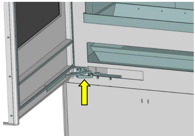
Fig. 21 : levier de blocage de la porte du foyer de combustion
