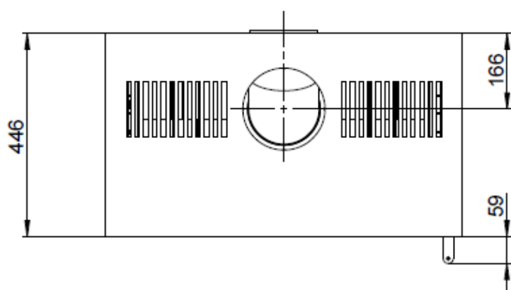
Fig. 2 : plan coté « myCastle » avec une rehausse
