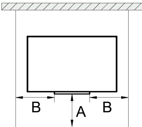
Fig. 6 Pare-étincelles
