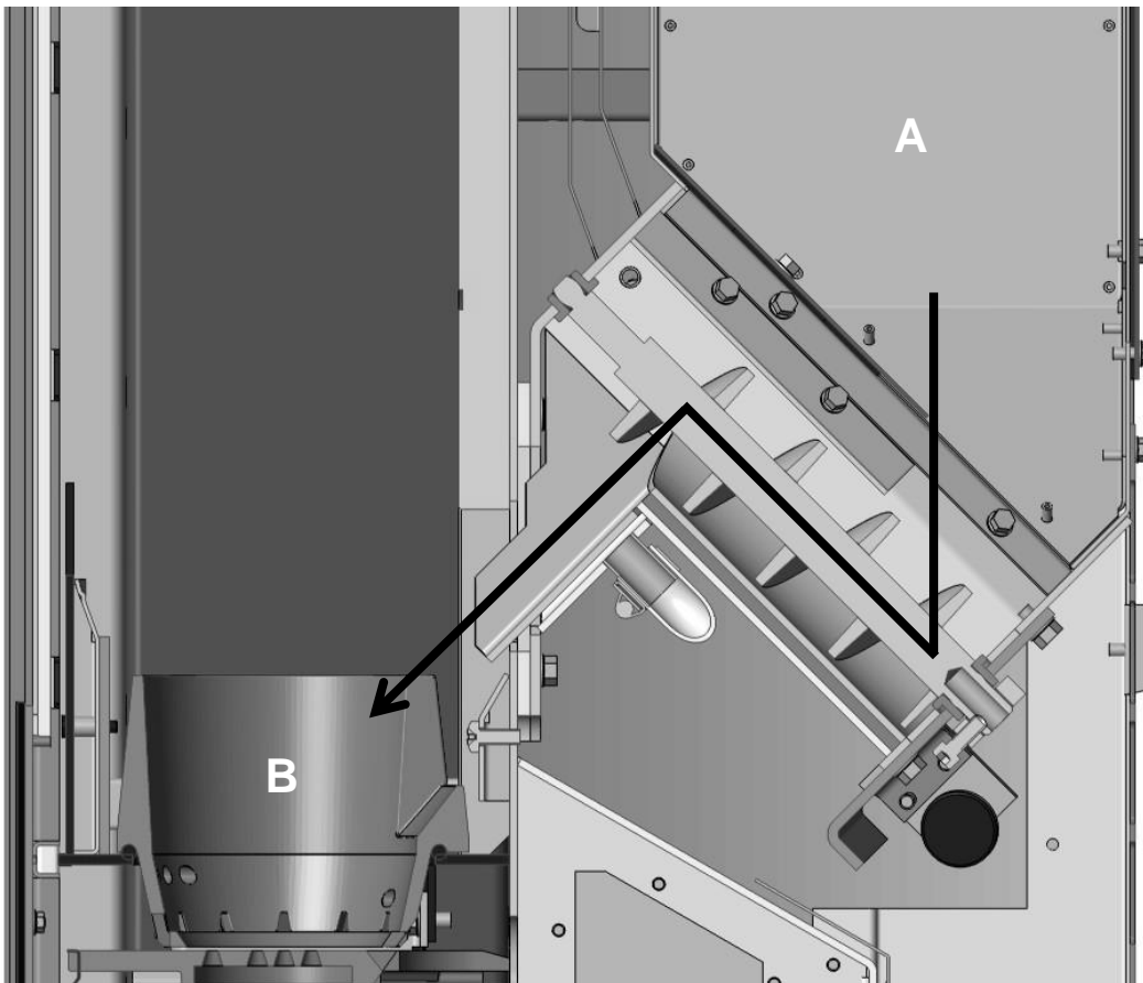
Fig. 64 : transport des pellets dans le PO 03
