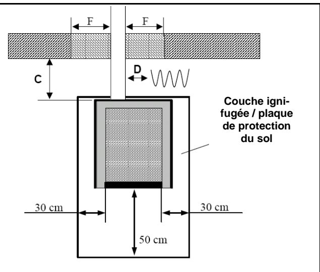
Exemple avec élément de raccordement à travers le mur avec des composants inflammables vers la cheminée
