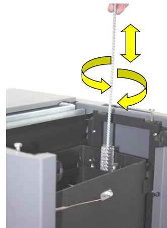
Fig. 86 : nettoyage des tirages de gaz de combustion
