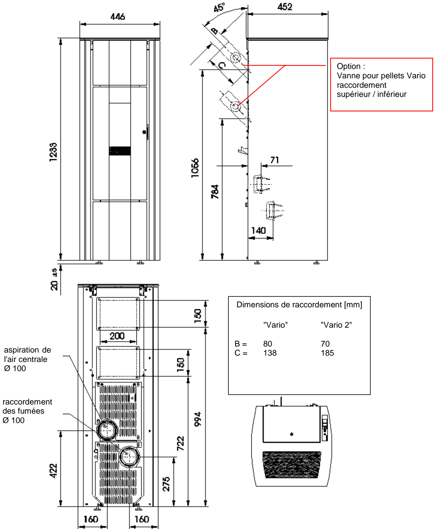
Fig. 99 : dessin coté PO 03
