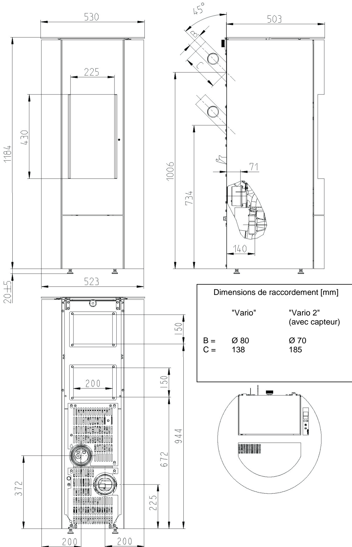
Fig. 101 : dessin coté PO 03-5
