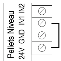
Fig. 47 : entrée Niveau Pellets
