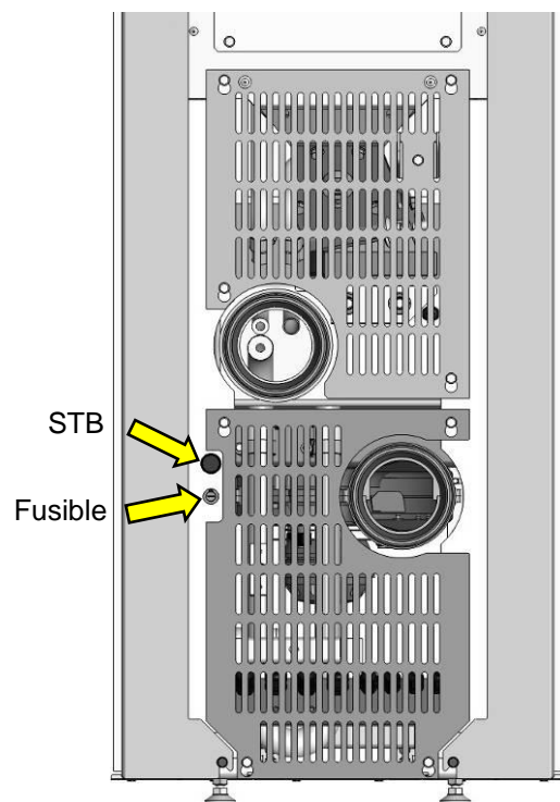
Fig. 57 : position STB et fusible
