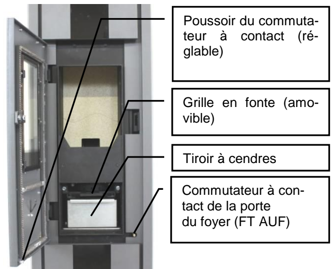
Fig. 67 : vue avant daily.nrg®
