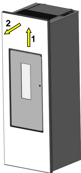
Fig. 16 : démontage de la vitre décorative frontale
