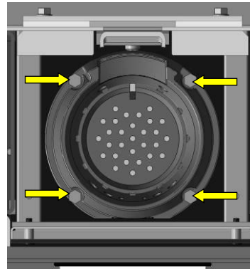
Fig. 80 : vissages pot brûleur
