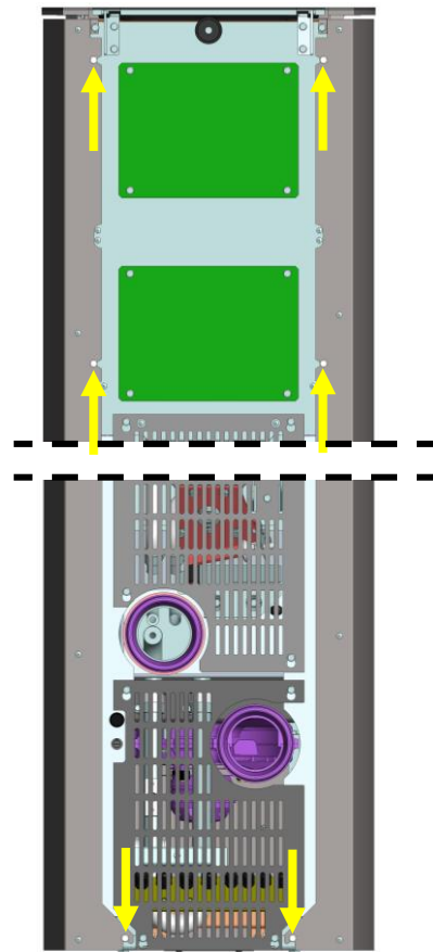
Fig. 10 : vue arrière daily.nrg®
