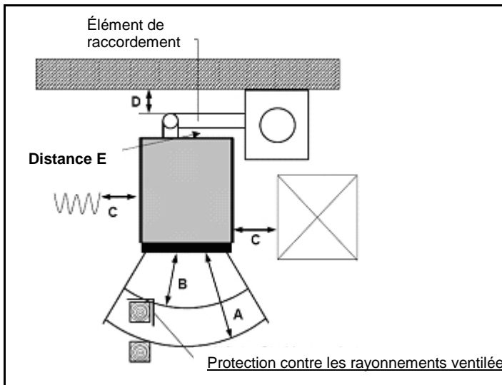
Exemple d'un élément de raccordement à la cheminée dans la pièce où se trouve l'appareil
