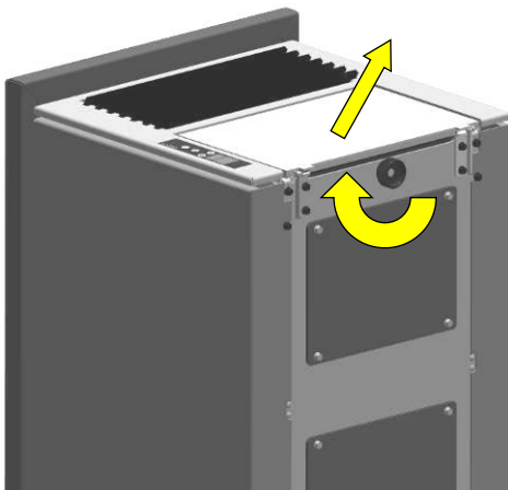
Fig. 60 : ouverture de la réserve de pellets
