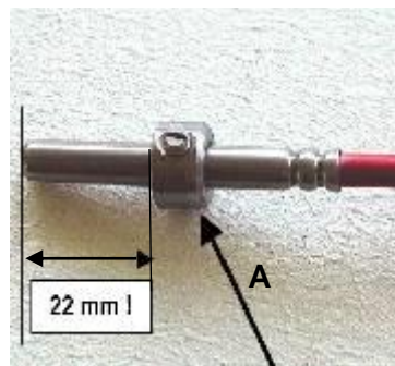
Fig. 58 : capteur TP
