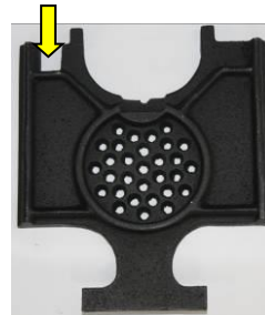
Fig. 74 : grille en fonte mal positionnée
