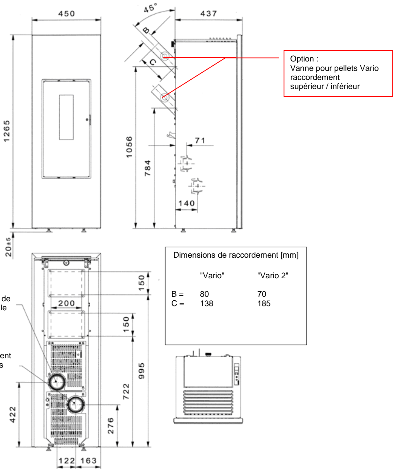
Fig. 100 : dessin coté PO 03-2
