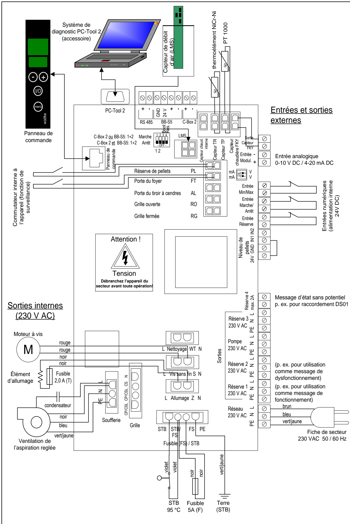
Fig. 36 : plan de câblage série PO 03
