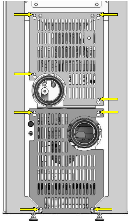
Fig. 14 : vue arrière série PO 03
