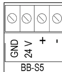
Fig. 45 : entrée Touch Control
