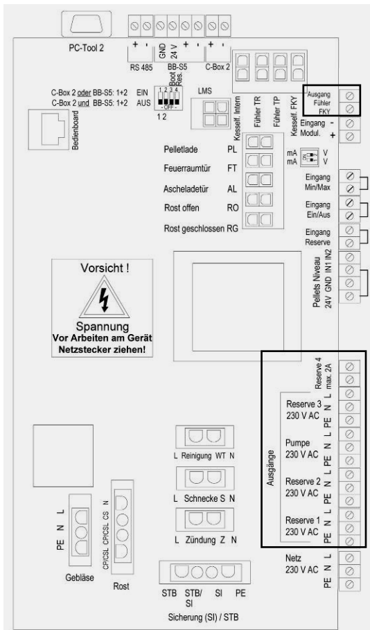
Fig. 49 : sorties carte-mère
