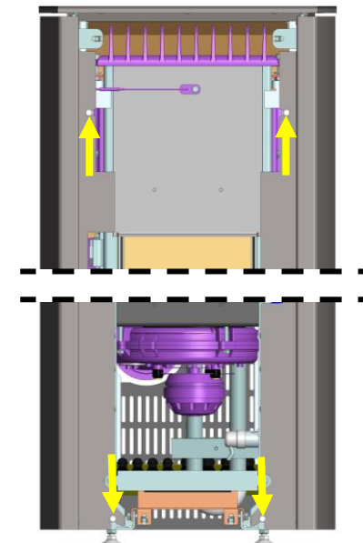
Fig. 11 : avant daily.nrg®
