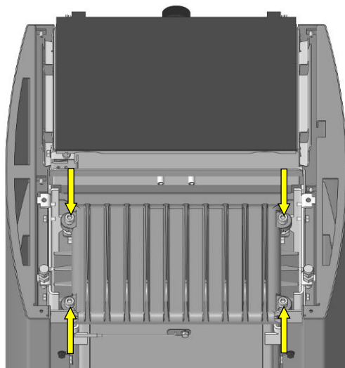
Fig. 83 : vis du couvercle en fonte
