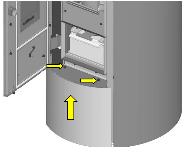
Fig. 26 : démonter l'habillage inférieur
