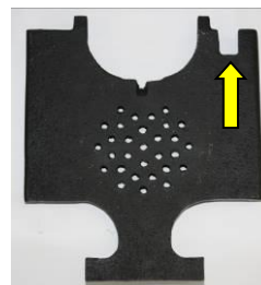
Fig. 75 : grille en fonte bien positionnée
