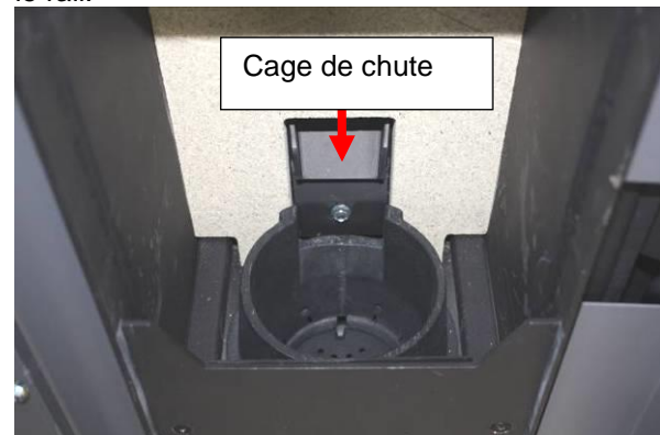
Fig. 97 : cage de chute des pellets
