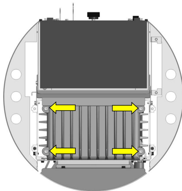
Fig. 92 : démontage du couvercle en fonte crazy.nrg
