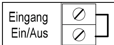
Fig. 38 : entrée Marche / Arrêt
