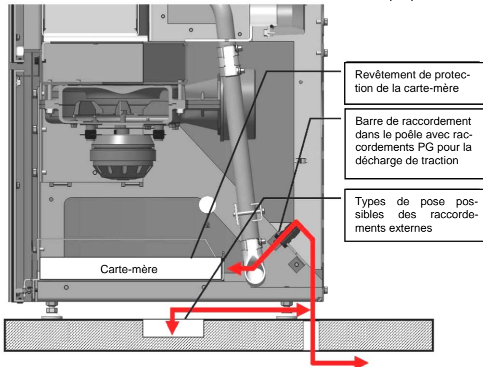
Fig. 32 : croquis de raccordement
