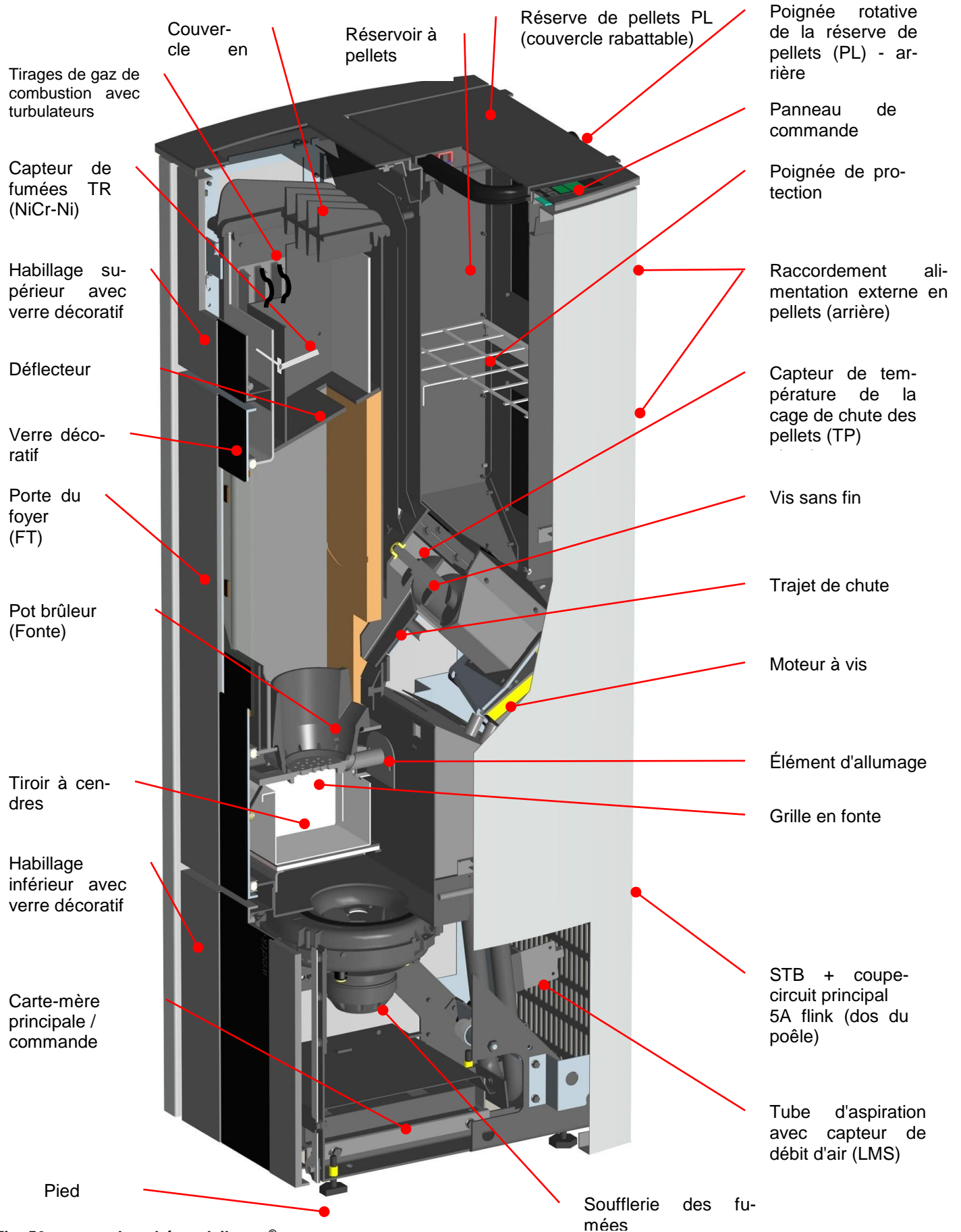
Fig. 56 : coupe du schéma daily.nrg®
