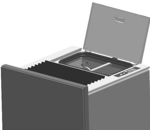
Fig. 61 : réserve de pellets ouverte
