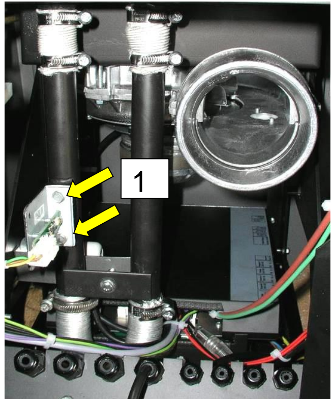
Fig. 96 : vissages du capteur de débit d'air
