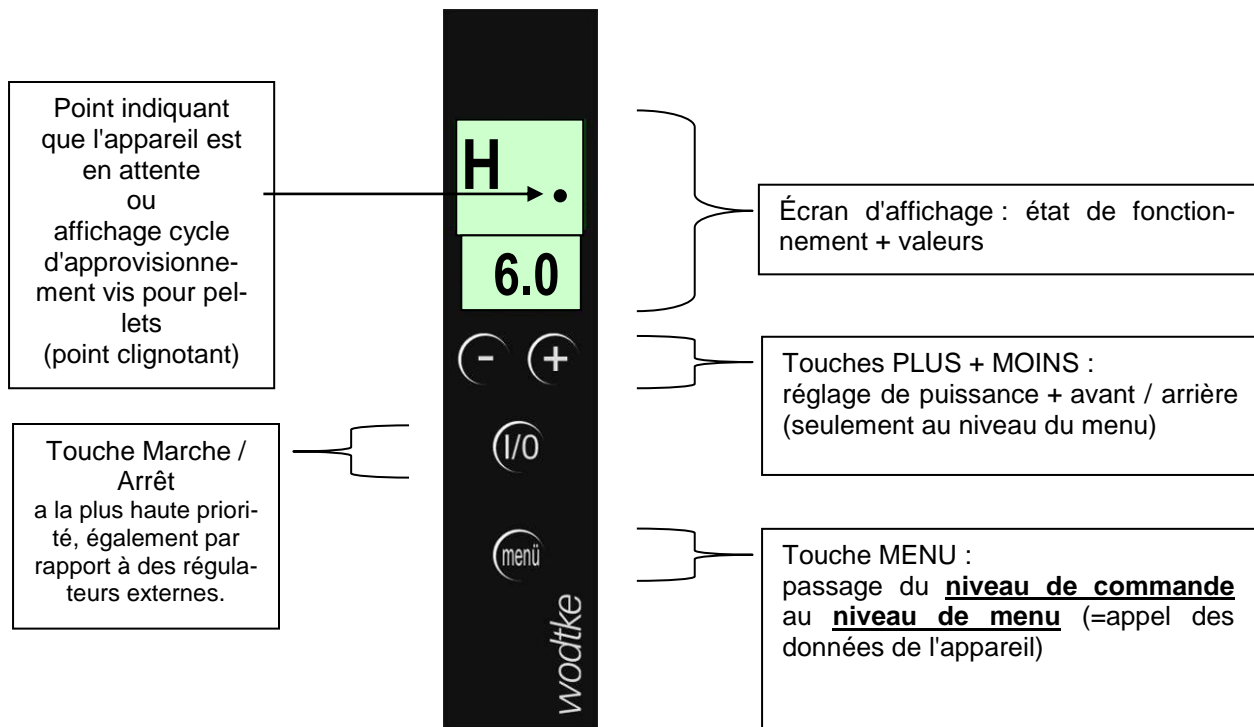
Fig. 66 : panneau de commande
