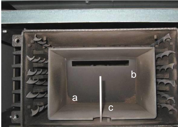
Fig. 87 : cendrier
