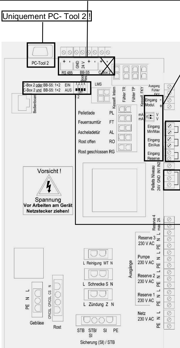
Fig. 37 : entrées carte-mère
