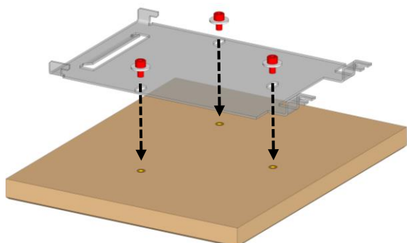
Fig. 6: raccorder le support avec les habillages avant
