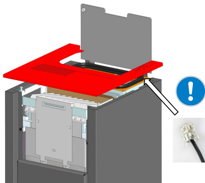
Fig. 2 : démontage du couvercle
