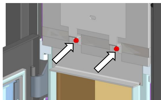
Fig. 4: vis de fixation de support du haut
