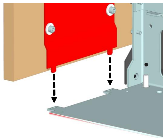
Fig. 8: positionner la paroi du bas
