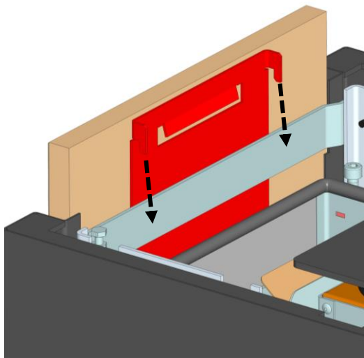
Fig. 7: accrocher la paroi du haut
